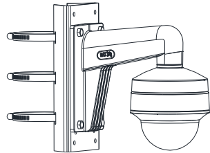
DS-1275ZJ-SUS Montage sur poteau vertical
